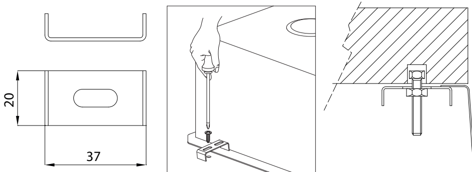
Крюк для моек под столешницей
